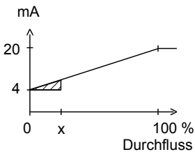
Stromausgang
